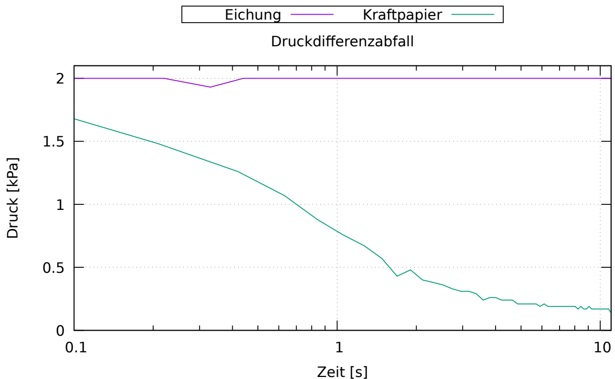
Abbildung 1: Druckdifferenzabfall der Probe im Vergleich zum Eichverlauf des Messplatzes
